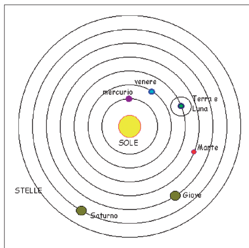
Il Cîl di Copernico e Galileo - il Soreli al è tal centri.
