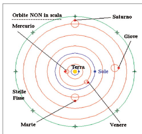
Il Cîl di Tolomeo - la Tere e je simpri tal centri e dut i zire ator.
