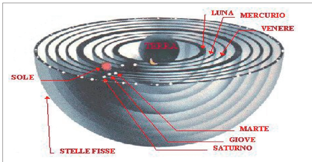
Il Cîl di Eudosso adotât ancje di Aristotele - la Tere e je tal centri des sferis concentrichis.
