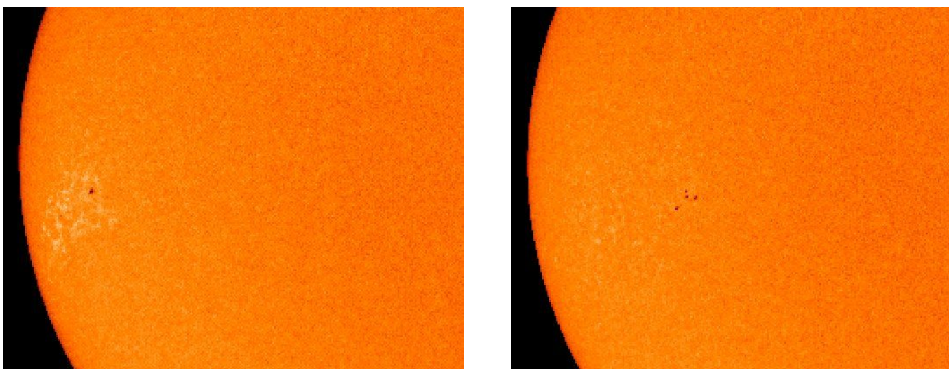
Immagine della sonda SOHO/MDI
